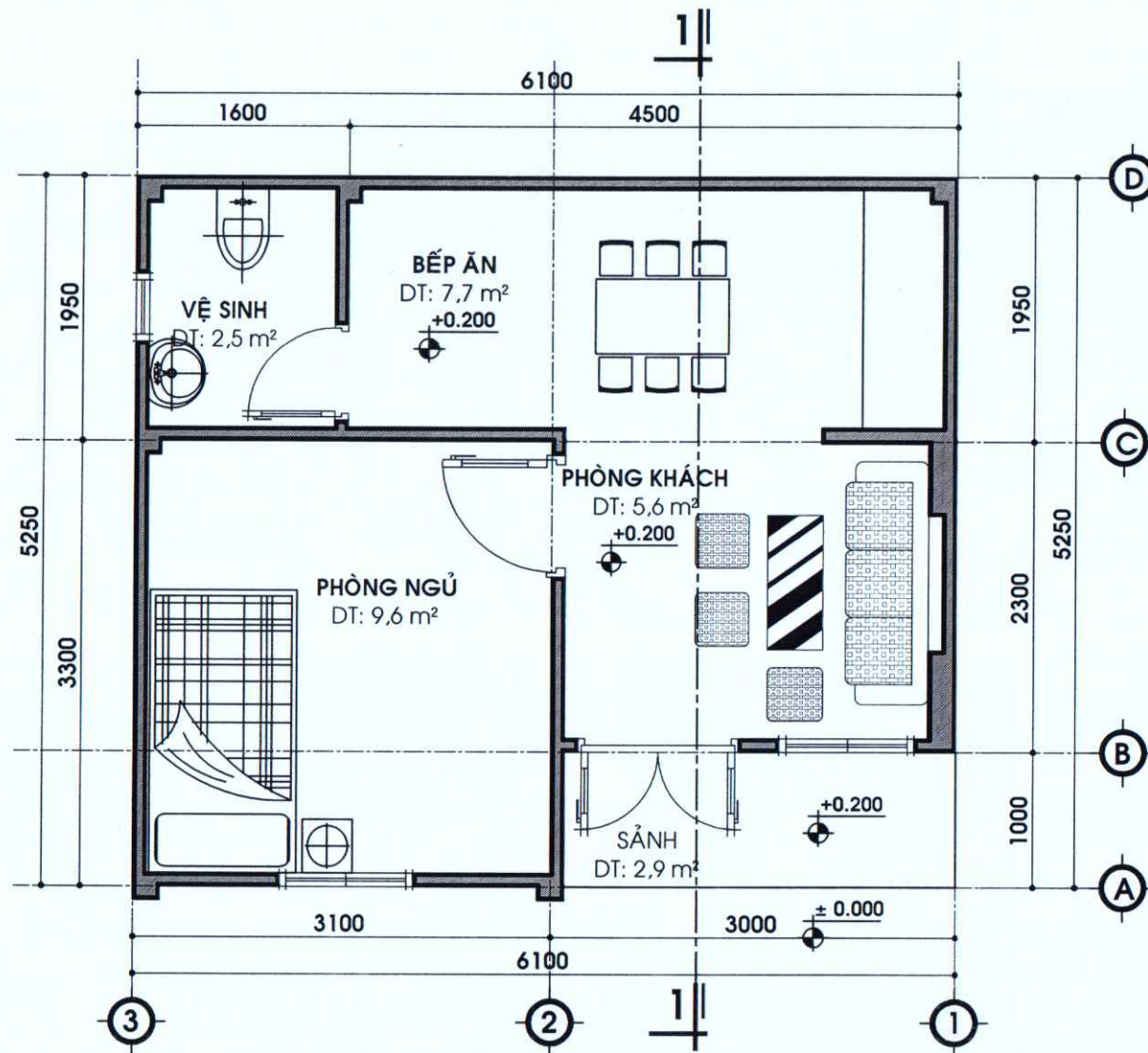
MẶT BẰNG NHÀ, TỶ LỆ: 1/50
