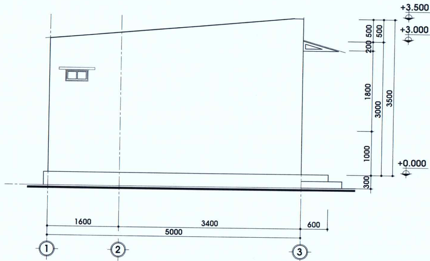
MẶT ĐỨNG TRỰC 1-3, TỶ LỆ: 1/50
