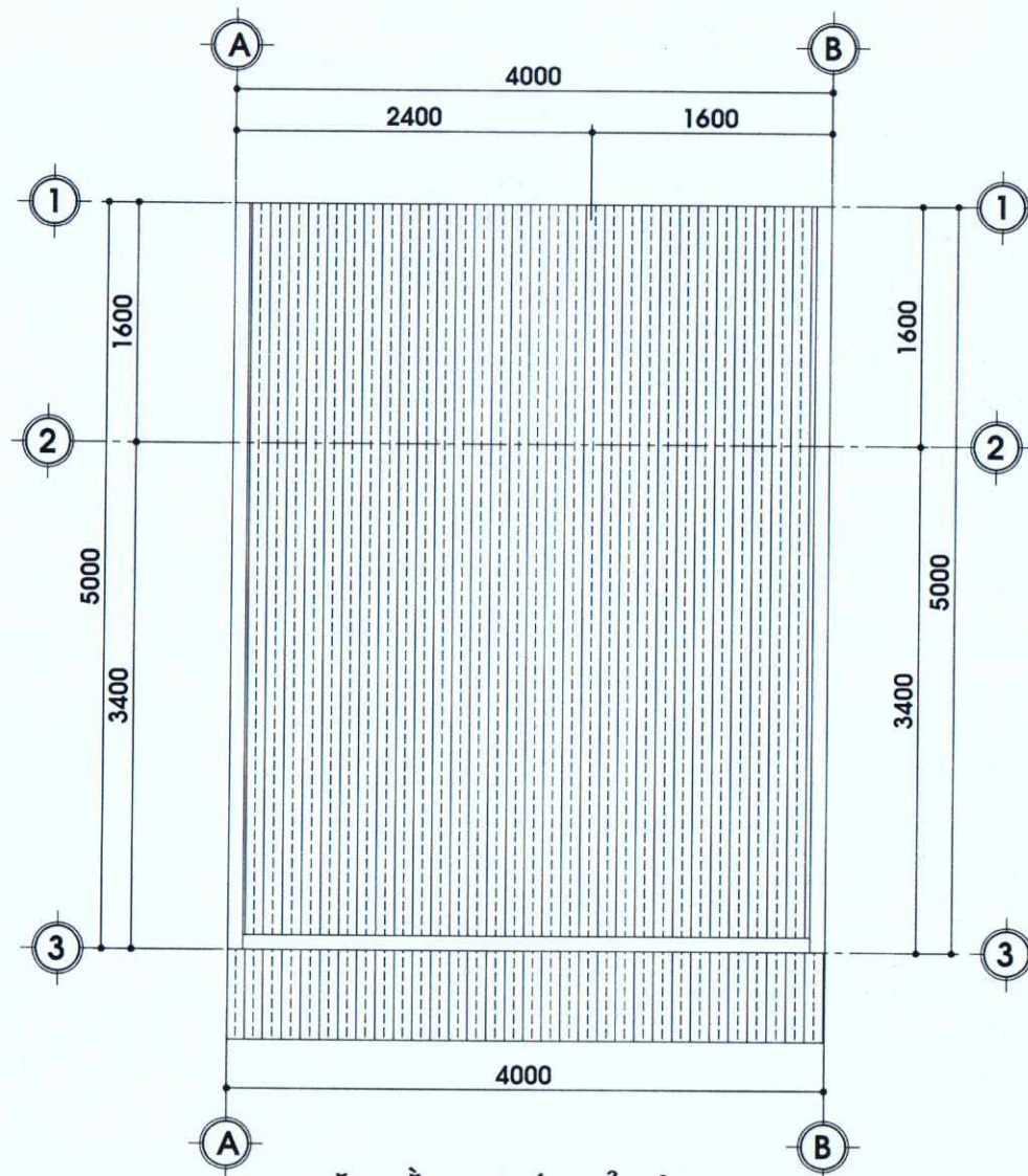
MẶT BẰNG MÁI, TỶ LỆ: 1/50
