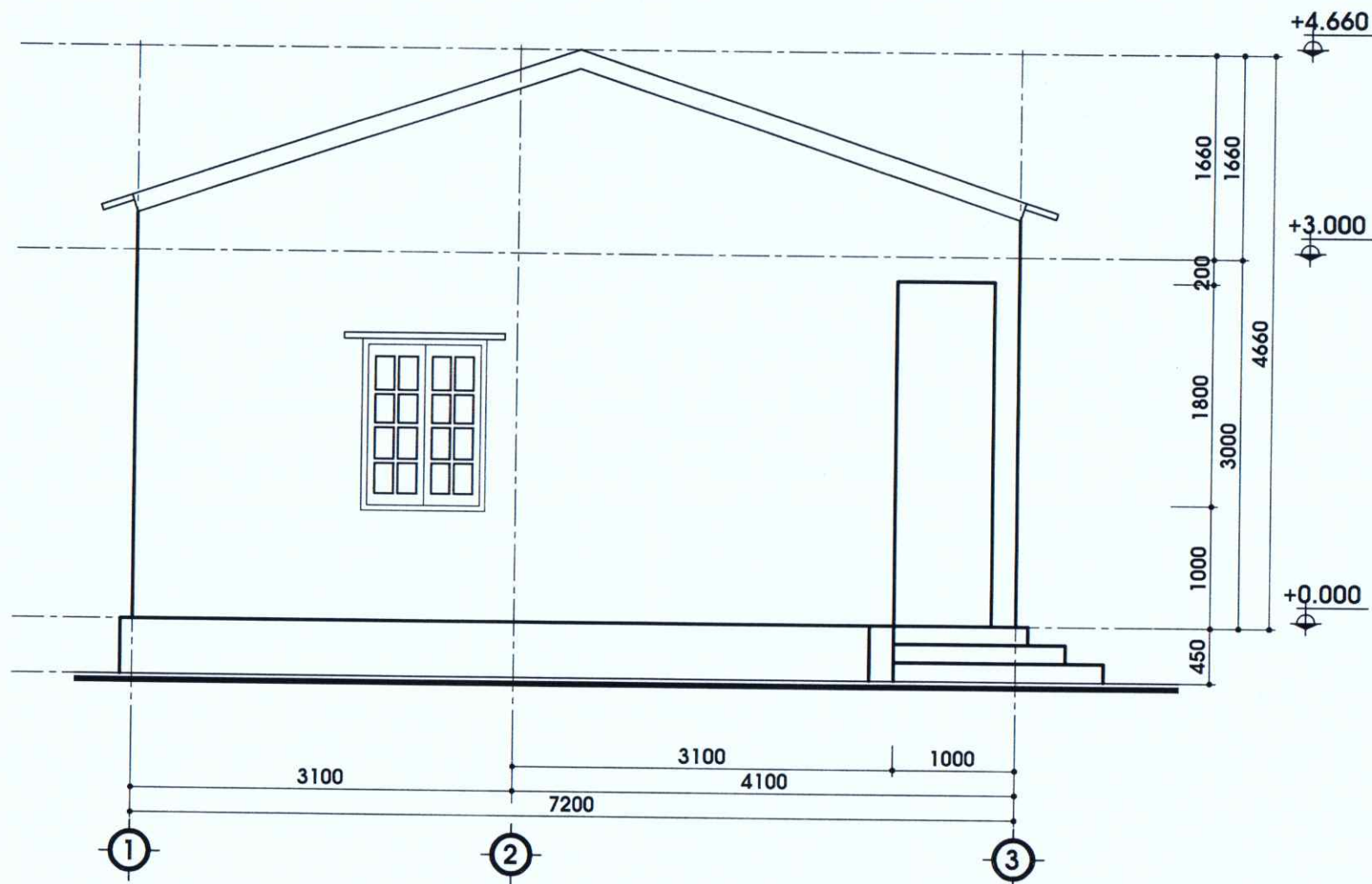
MẶT ĐỨNG TRỰC 1-3, TỶ LỆ: 1/50
