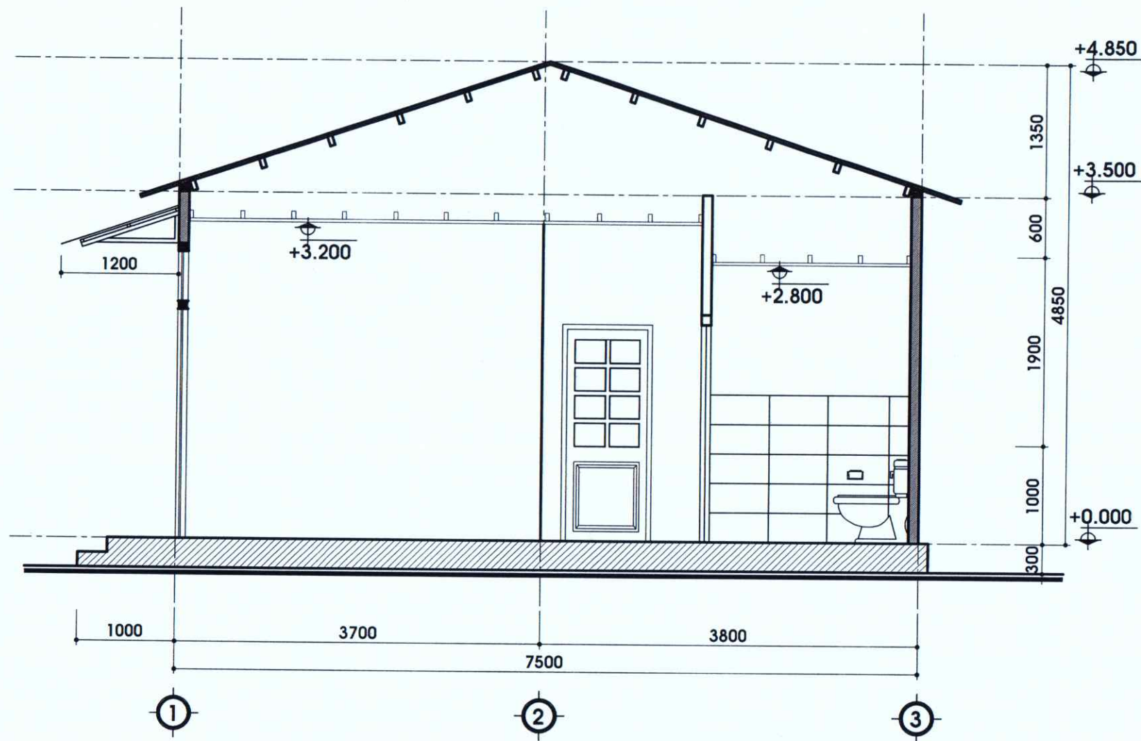
MẶT CẮT 1 - 1, TỶ LỆ: 1/50
