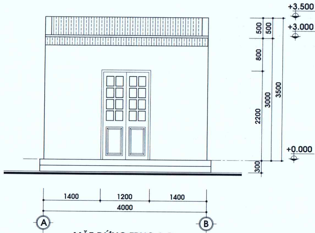
MẶT ĐỨNG TRỰC A-B, TỶ LỆ: 1/50
