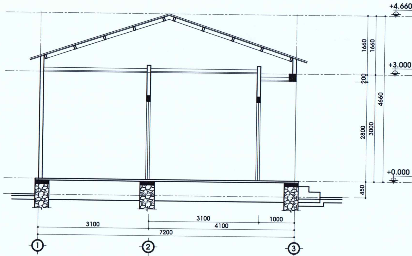
MẶT ĐỨNG TRỤC 1-3, TỶ LỆ: 1/50
