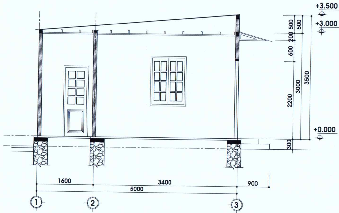
MẶT CẮT 1-1, TỶ LỆ: 1/50
