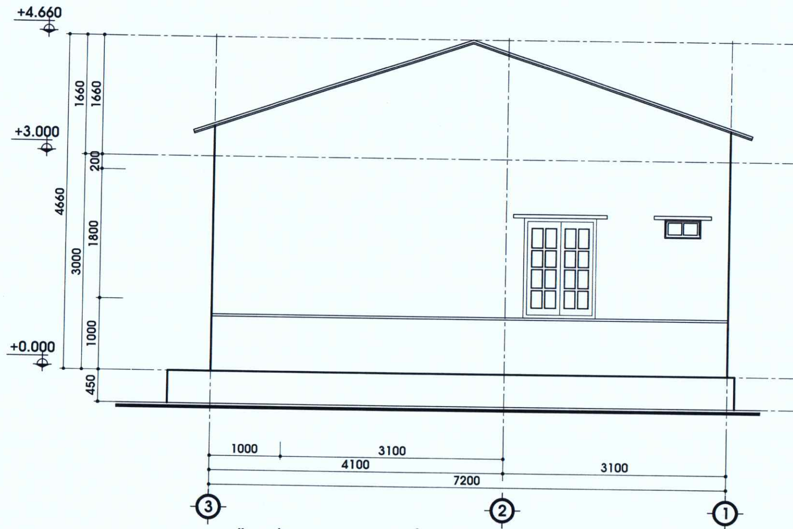
MẶT ĐỨNG TRỰC 3-1, TỶ LỆ: 1/50
