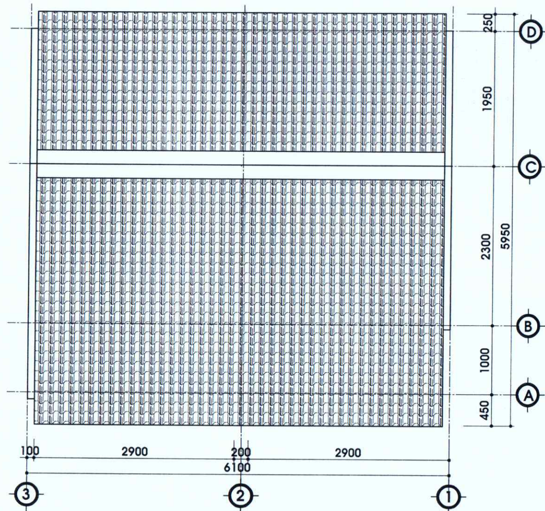
MẶT BẰNG MÁI, TỶ LỆ: 1/50
