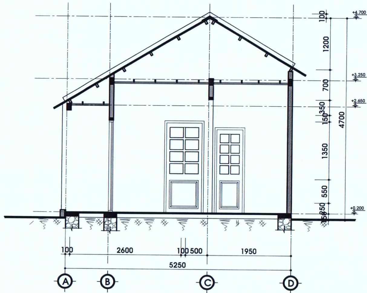
MẶT CẮT 1 - 1, TỶ LỆ: 1/50
