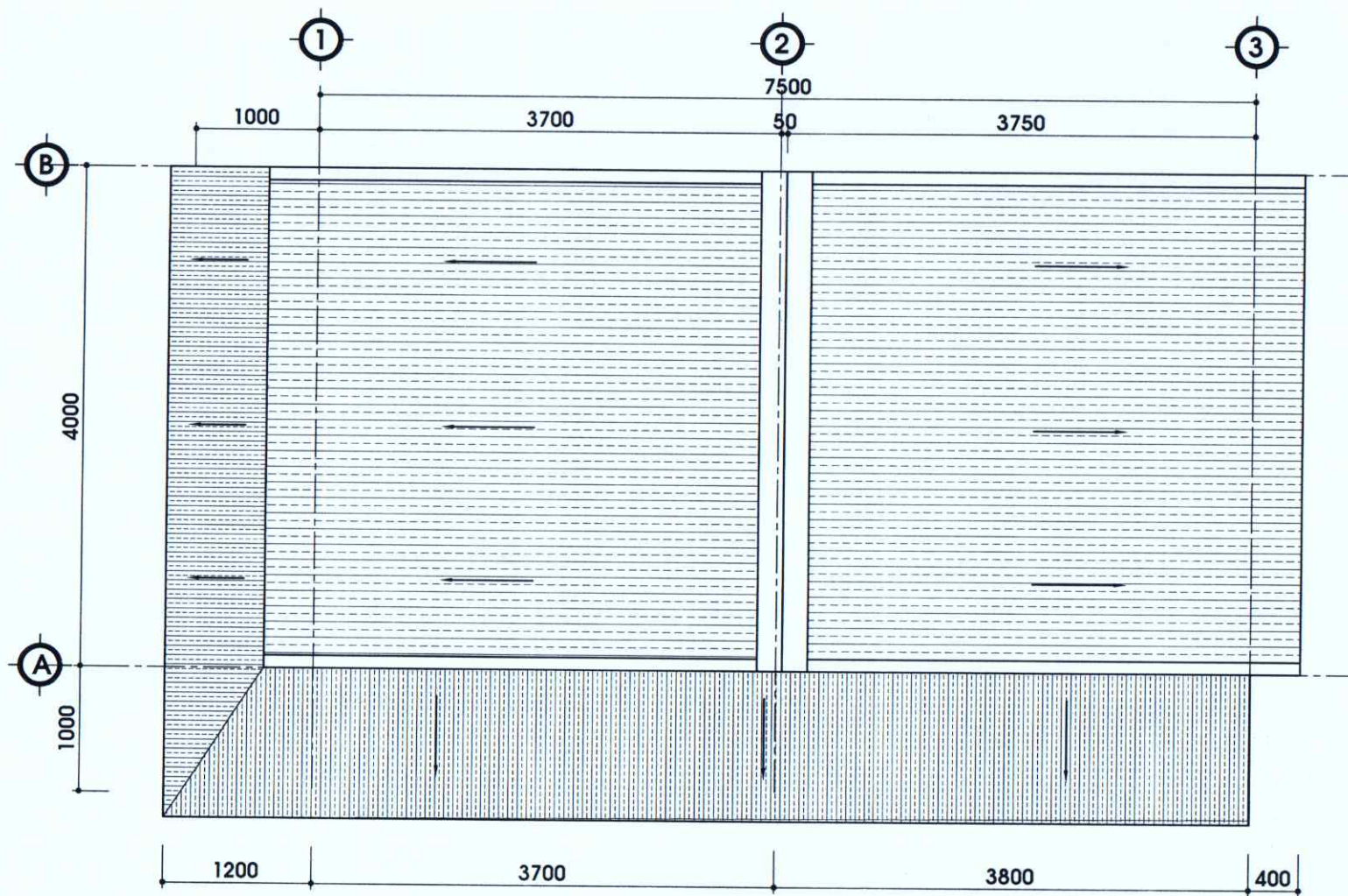
MẶT BẰNG MÁI, TỶ LỆ: 1/50
