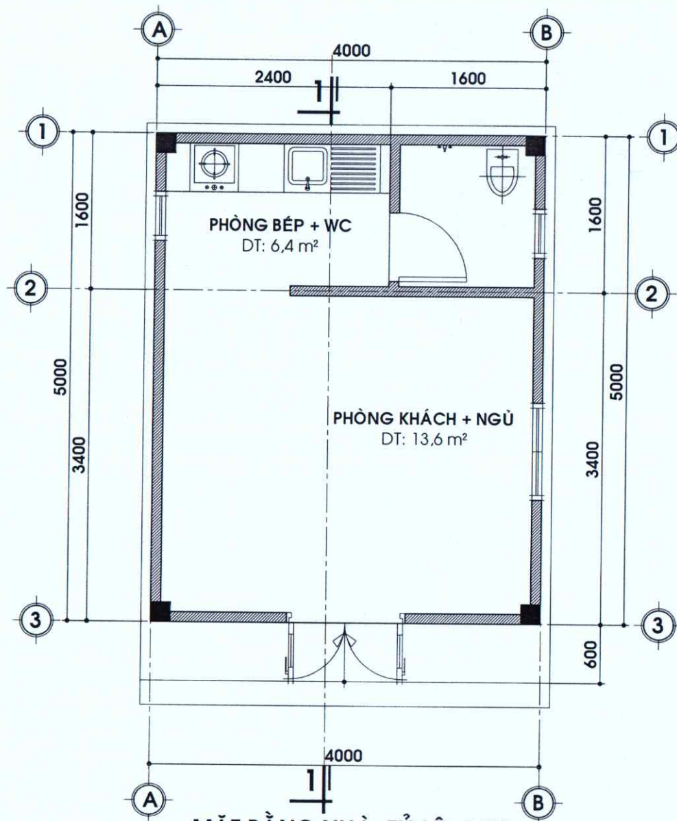
MẶT BẰNG NHÀ, TỶ LỆ: 1/50
