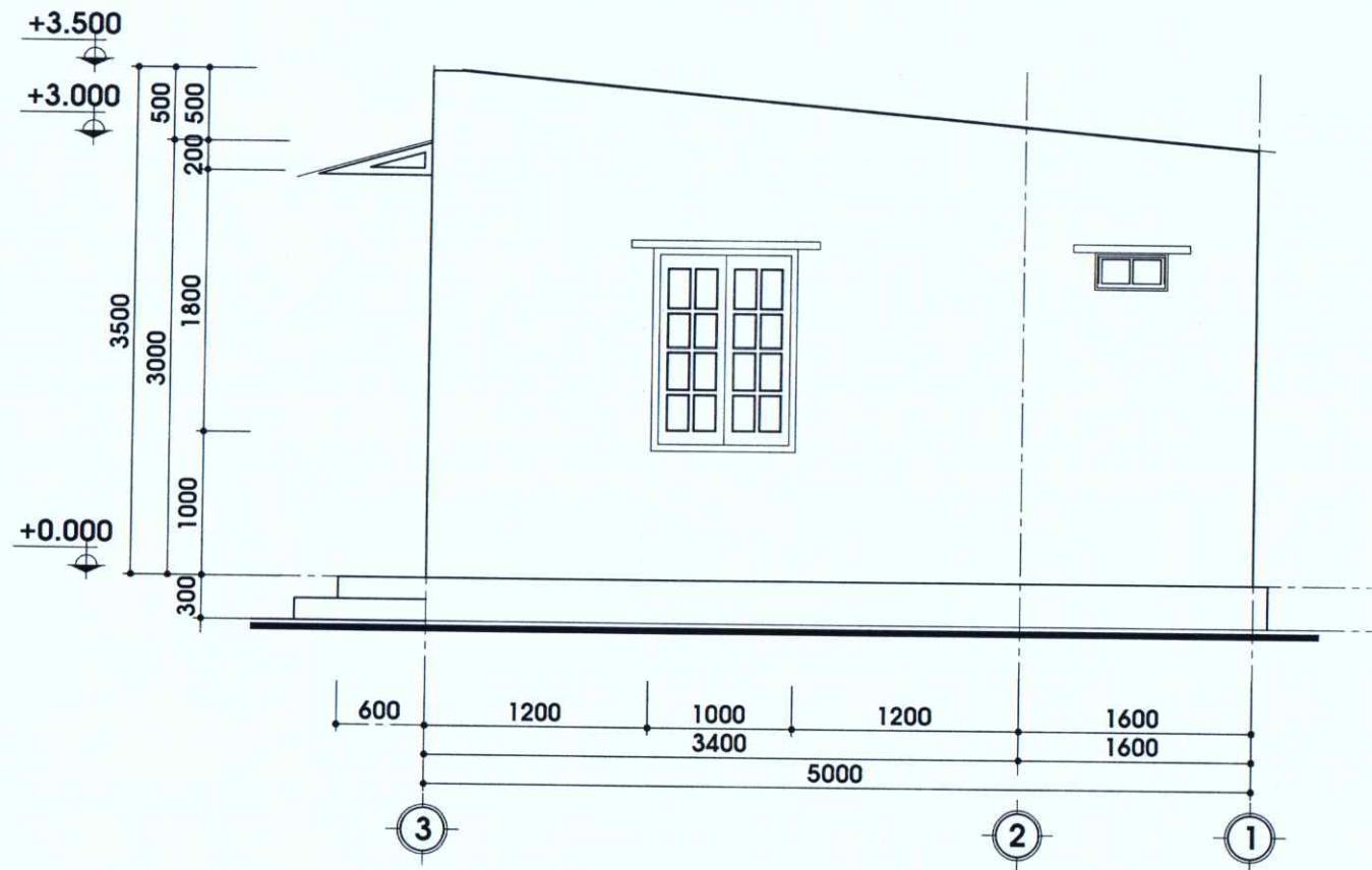
MẶT ĐỨNG TRỰC 3-1, TỶ LỆ: 1/50
