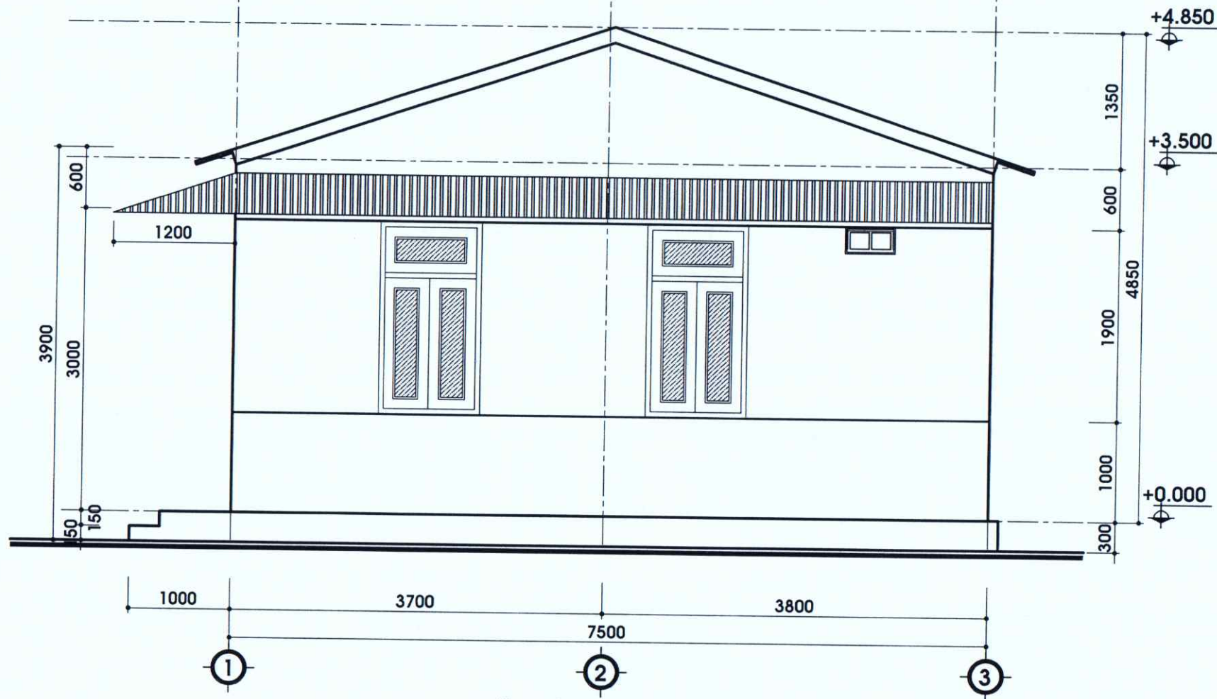
MẶT ĐỨNG TRỰC 1-3, TỶ LỆ: 1/50
